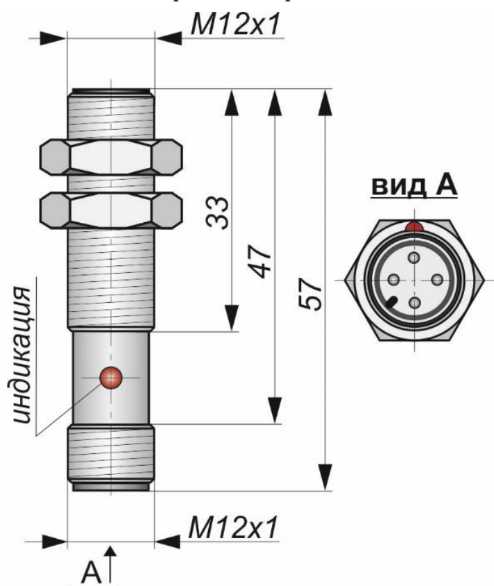
Габаритный чертеж
